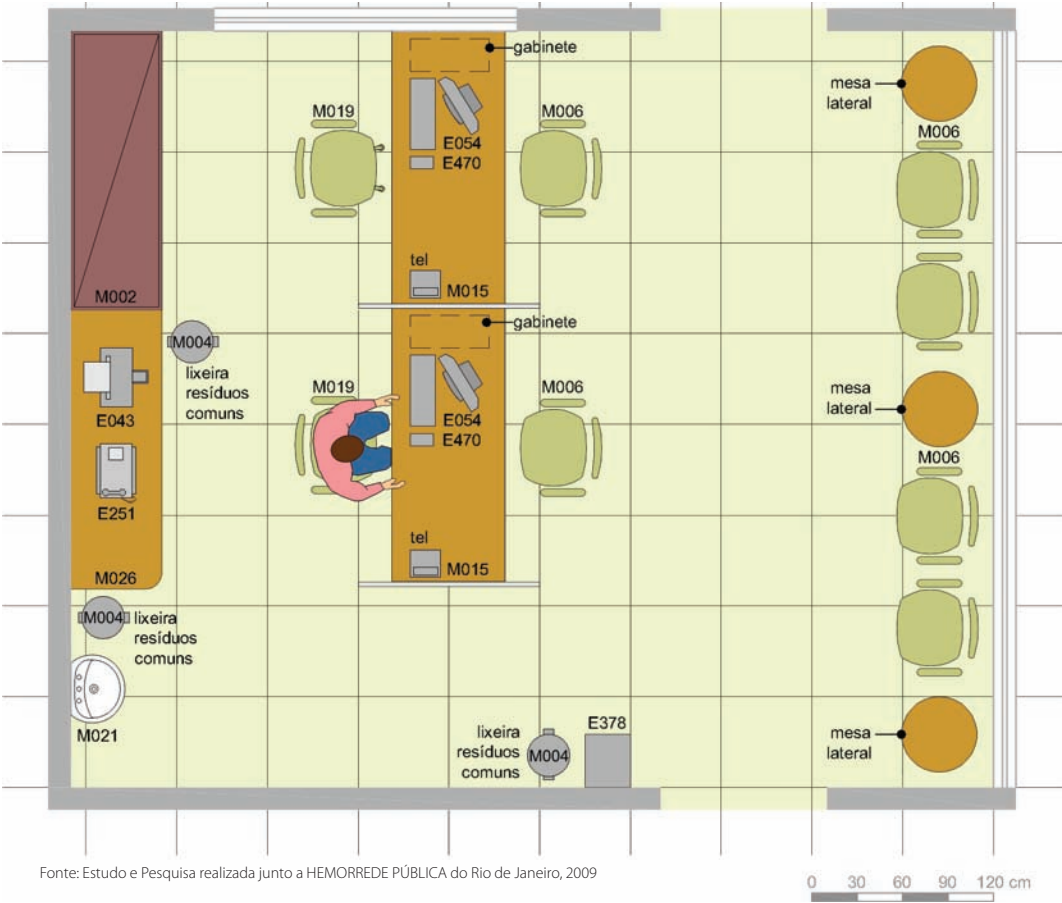
Figura 49: Layout.
